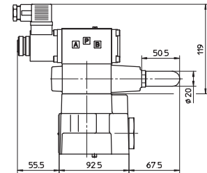
AGIU-10/**-IX; Масса = 5,3 кг
