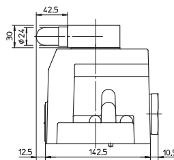
AGIR-32; Масса = 9,4 кг AGIRR-32; Масса = 9,6 кг
