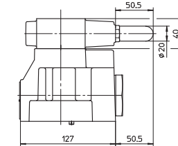
AGIS-20; Масса = 6 кг AGISR-20; Масса = 6,2 кг AGIU-20; Масса = 6 кг
