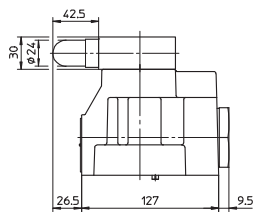
AGIR-20; Масса = 5,5 кг AGIRR-20; Масса = 5,7 кг
