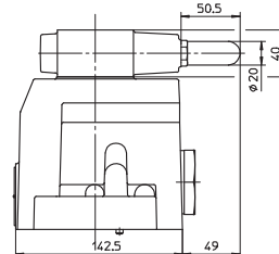
AGIS-32; Масса = 9,9 кг AGISR-32; Масса = 10,1 кг AGIU-32; Масса = 9,9 кг
